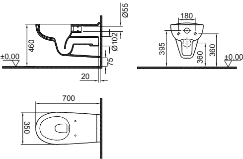
Technische Zeichnung
