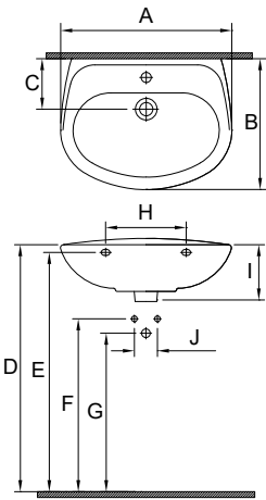
Technische Zeichnung
