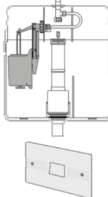
Mod. 81./80.000 1978 – 1983, P-IX 2171/I Mechanische Betätigung von vorne
