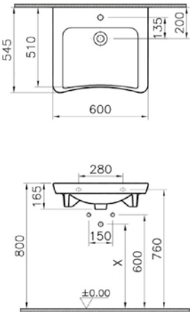
Technische Zeichnung
