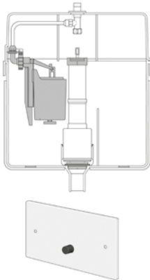
Mod. 81.000 1973 – 1976, P-IX 2171/I Mechanische Betätigung von vorne
